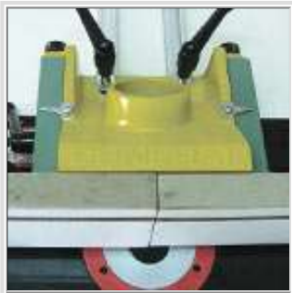
Rails de guidage du guide
